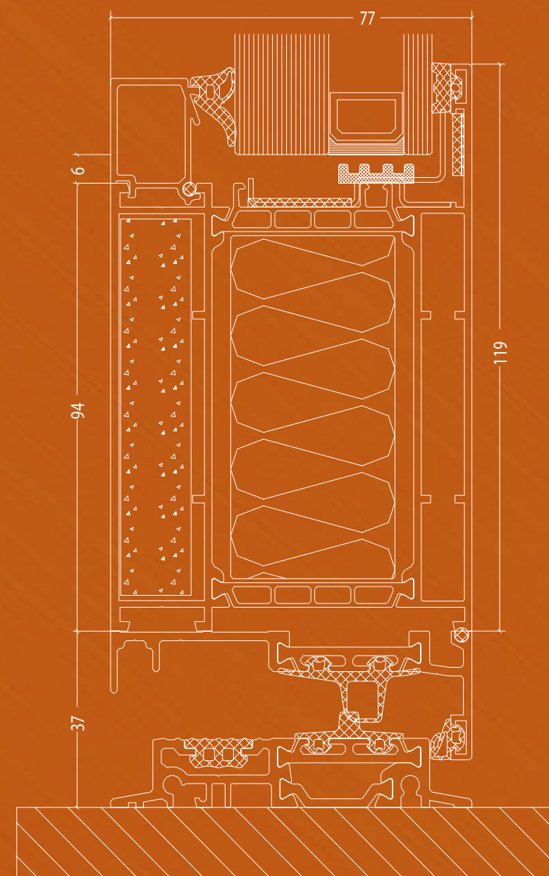
MB-86 EI 30 / DOOR /
