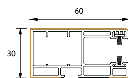
coulisse simple
