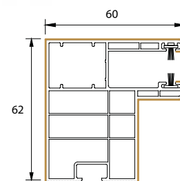
coulisse déportée
