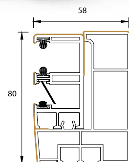
coulisse simple avec moustiquaire
