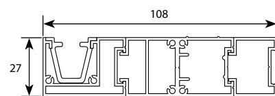
Coulisse simple avec déport
