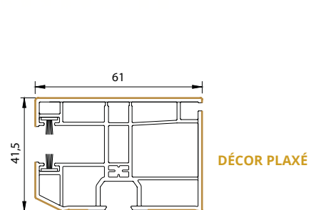
coulisse simple
