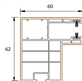
coulisse déportée
