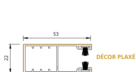
coulisse simple
