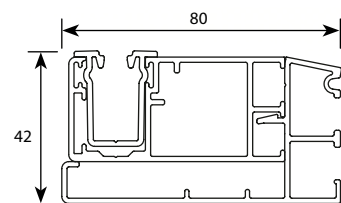
Coulisse simple
