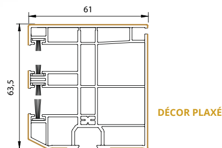
coulisse simple avec moustiquaire
