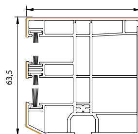
coulisse simple avec moustiquaire
